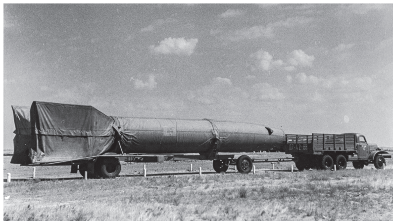
Vidutinio nuotolio branduolinė raketa R-2
